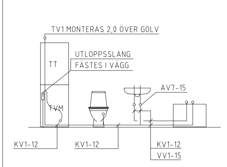
TYPRITNING BADRUM VATTENINSTALLATION
