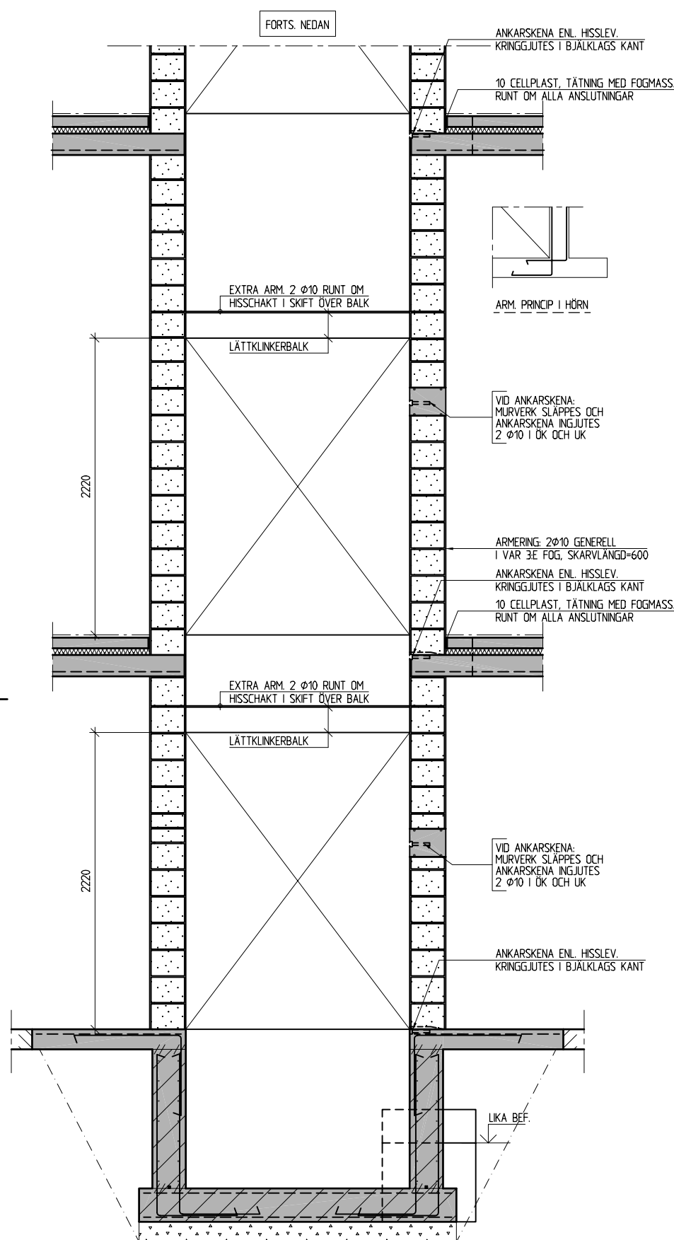
A 1:20 HISSGRÖP ENL. K320:11 TOMRÖR OCH INGJUTNINGSGODS FÖR HISS ENL. HISSLEVERANTÖR
